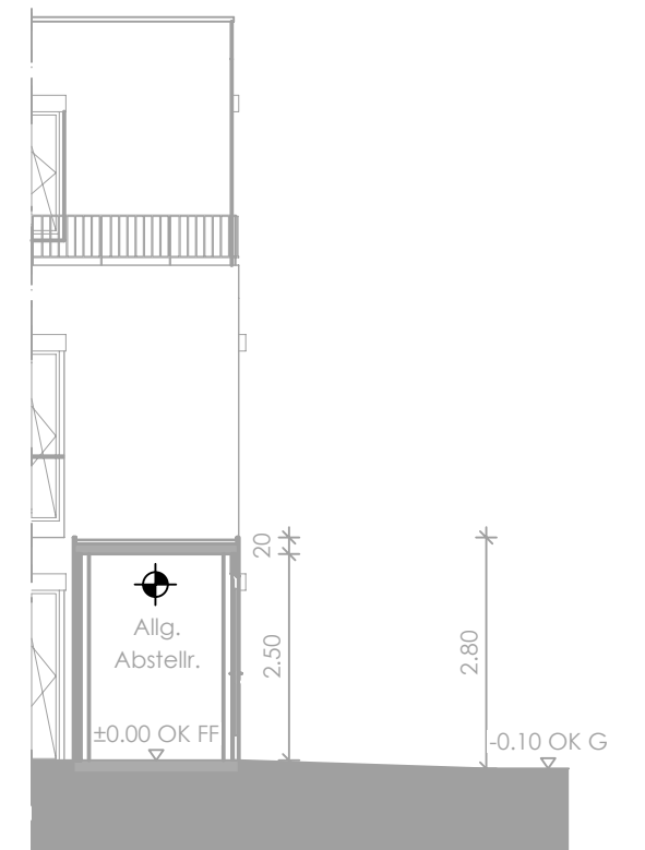
Schnitt C-C
