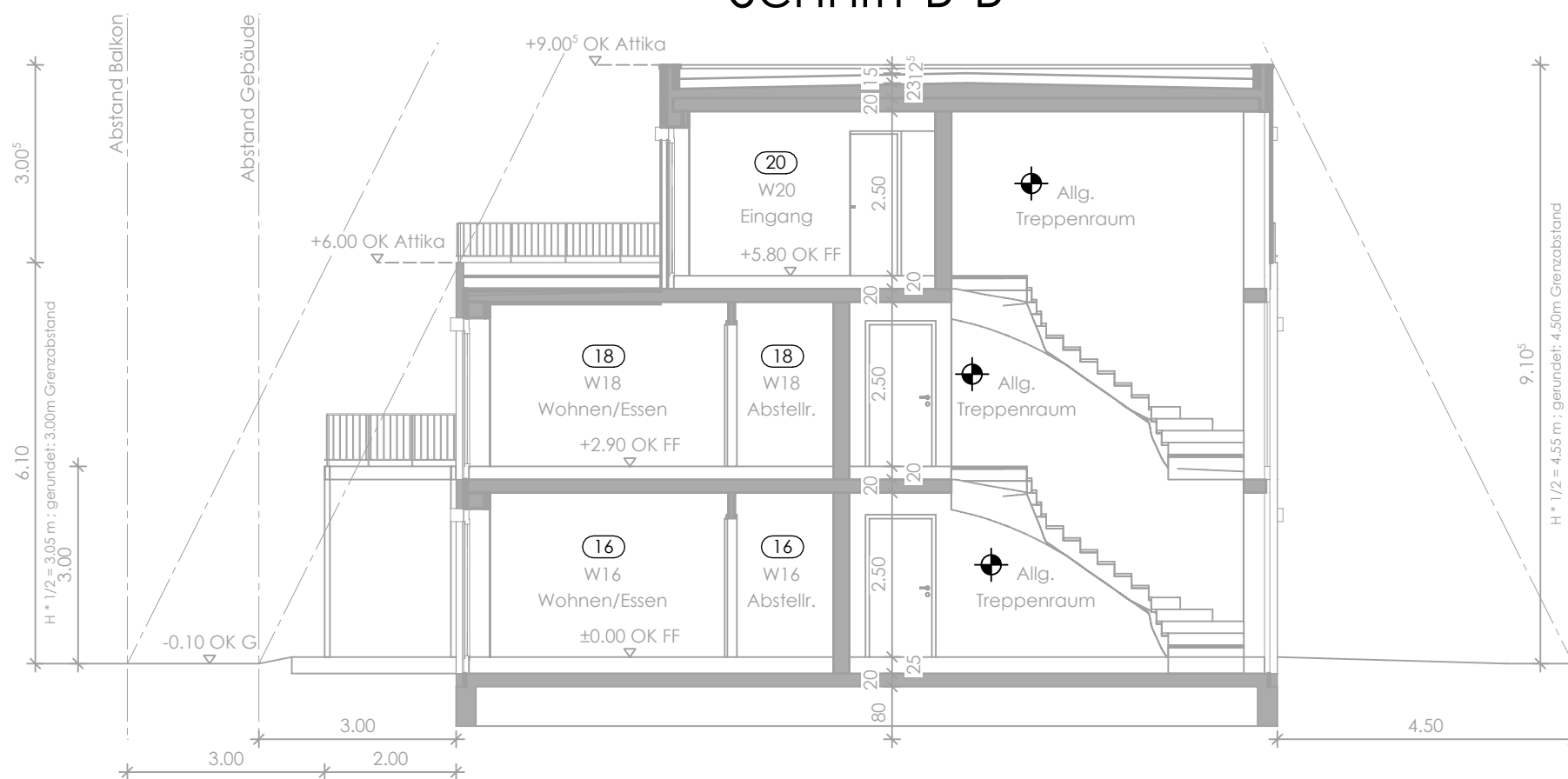
Schnitt B-B
