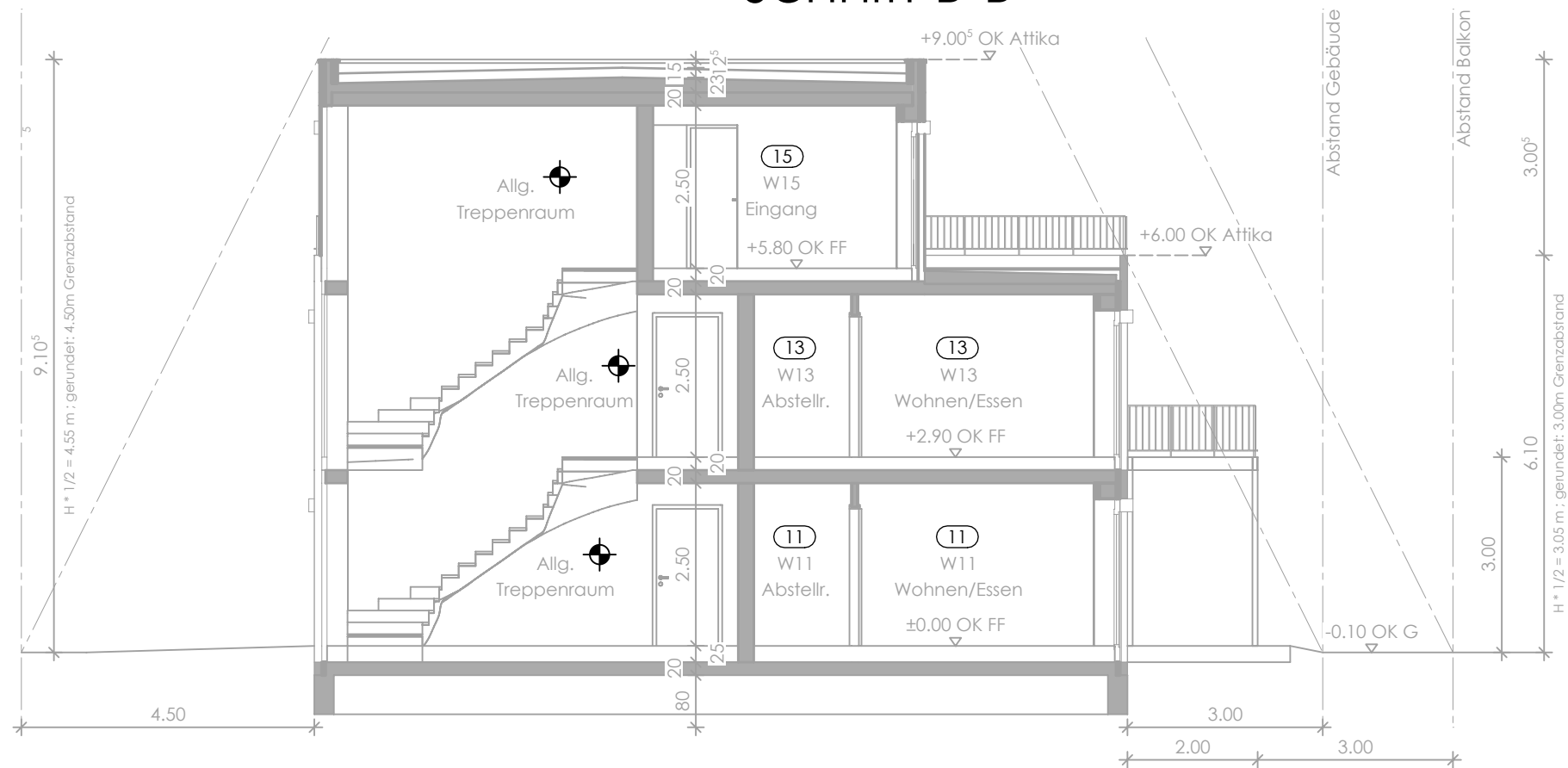
Schnitt B-B
