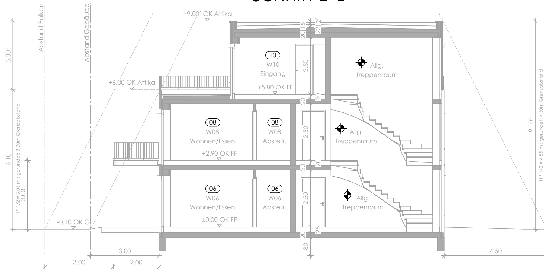
Schnitt B-B
