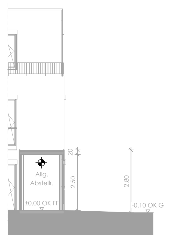
Schnitt C-C
