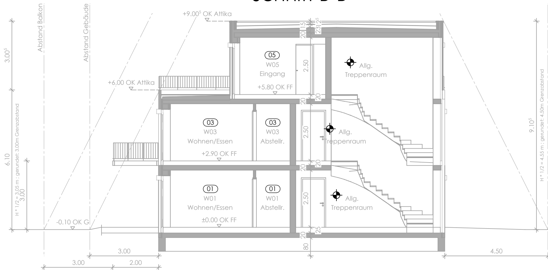
Schnitt B-B
